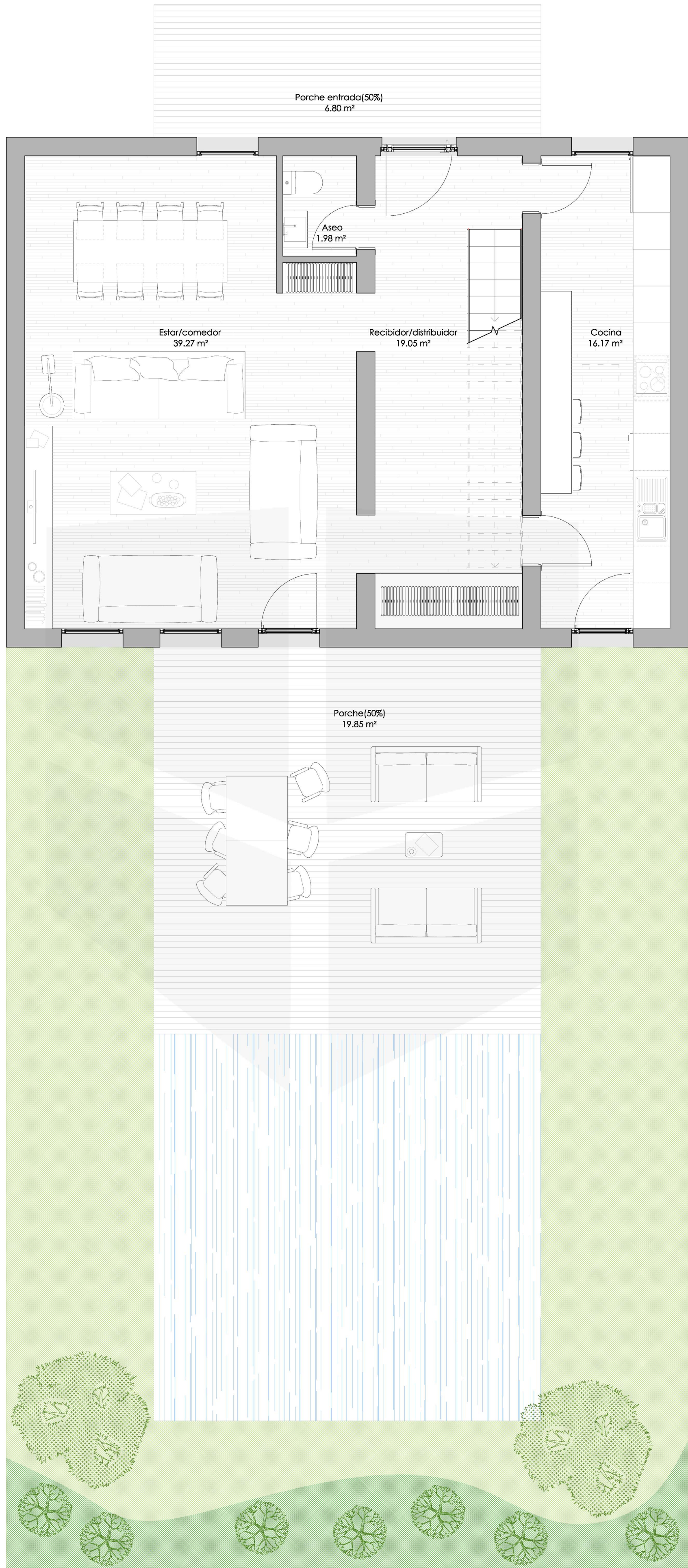
PLANTA BAJA E:1/50
